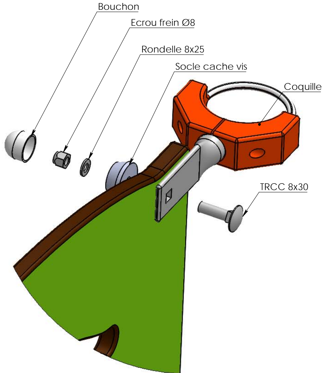
Détail A ECHELLE 1 : 2
