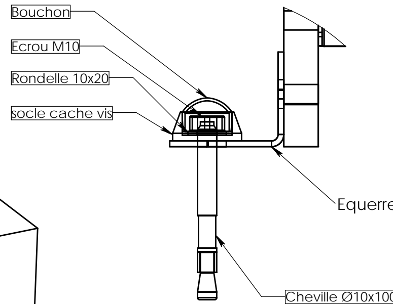
Fixation sur dalle béton par 4 chevilles Ø10x100
