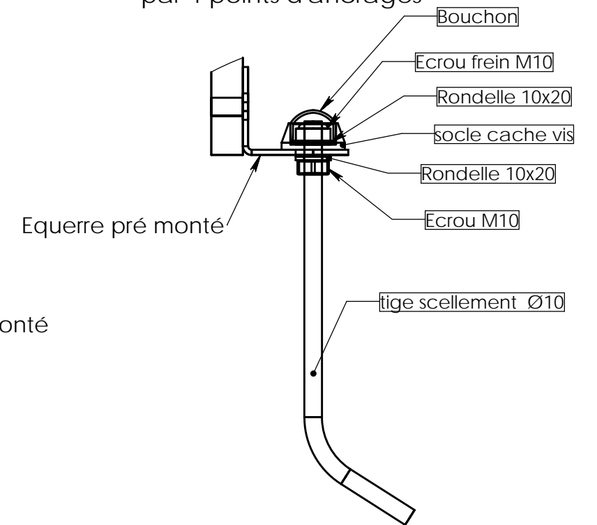
Fixation sur enrobé par 4 points d'ancrages
