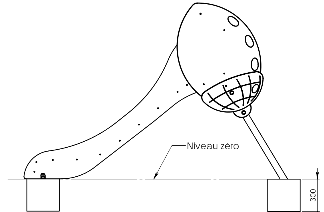
Fixation sur enrobé par 4 points d'ancrages
